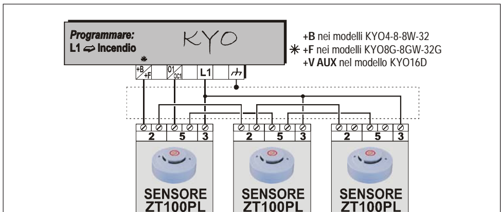
Fig. 2.8b - Collegamento di tre sensori Antincendio modello BENTEL ZT100PL (Fumo)
